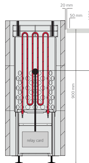
Abb. 5 Befestigung des Saunaofens am Fußboden
